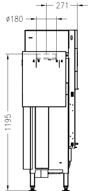
Seitenansicht M~1:20
